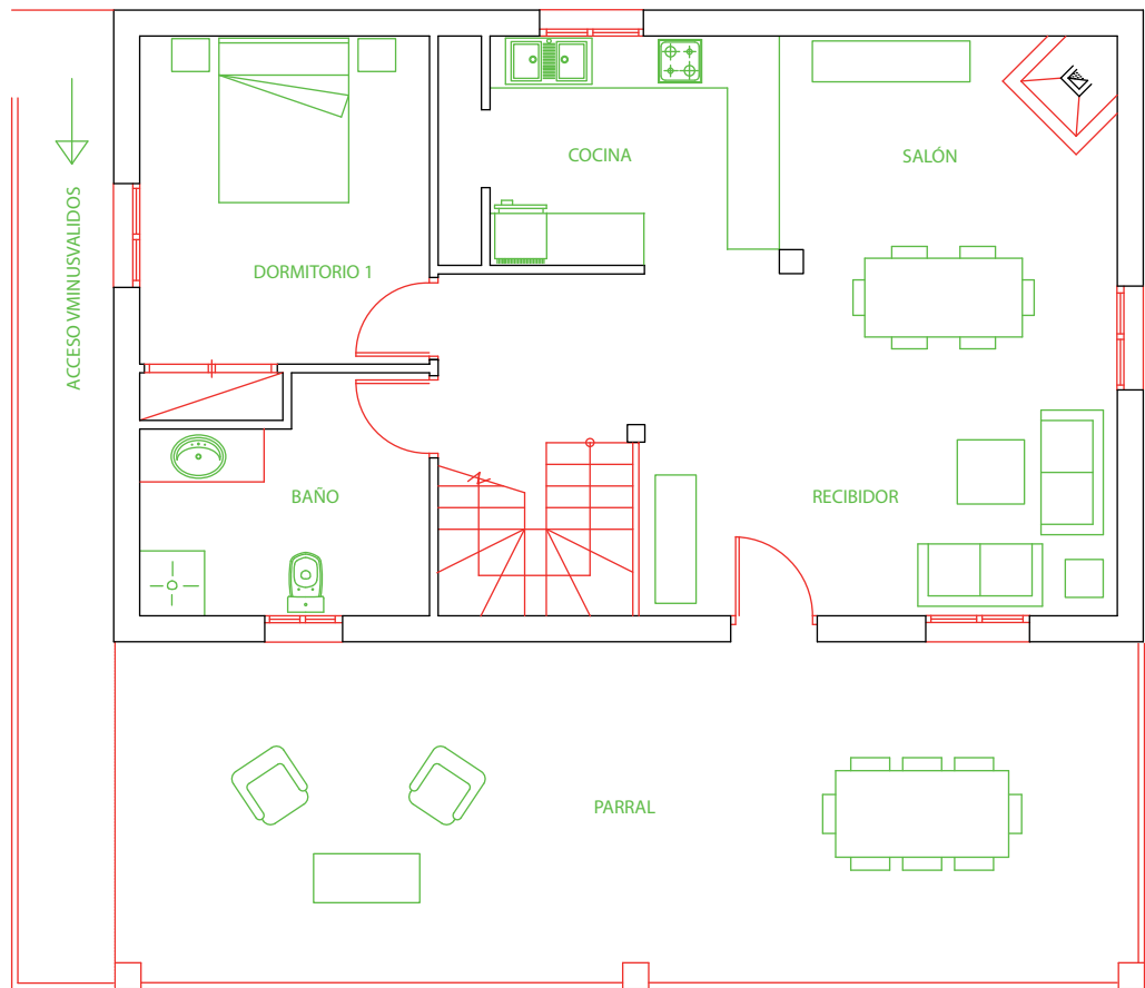
PLANTA BAJA
